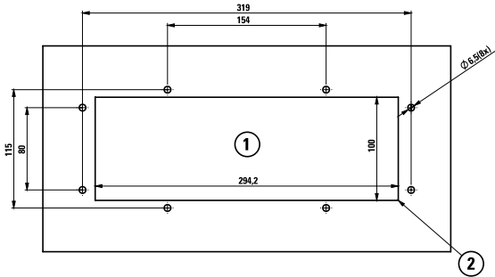
FIELDLED EVO 280_96 Einbau
